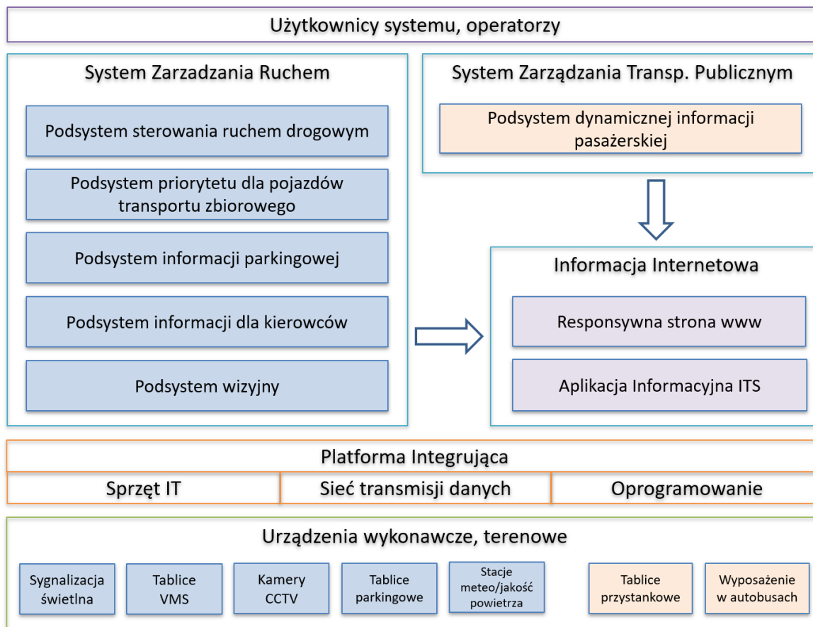
Rysunek 1. Architektura Systemu Zarządzania Ruchem w Świnoujściu
