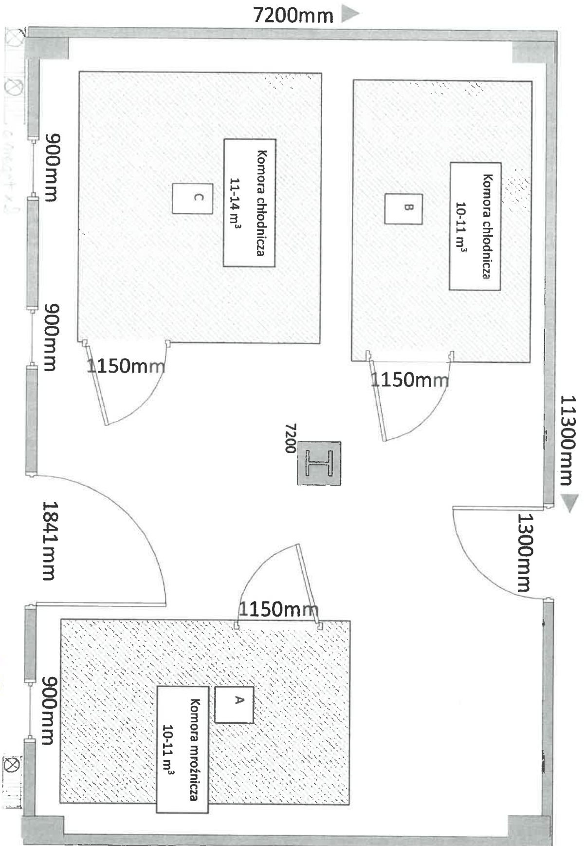
Rysunek nr 1. Magazyn żywnościowy – proponowane rozmieszczenie komór chłodniczych i mroźniczej.
