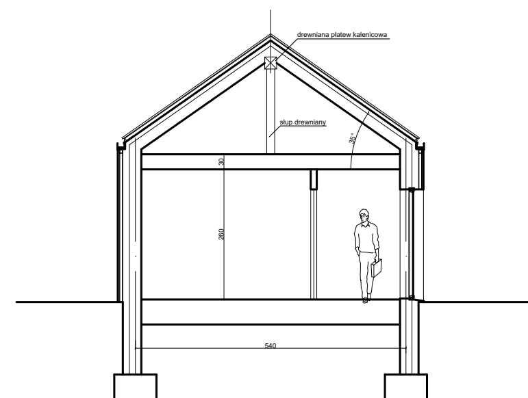
PRZEKRÓJ SCHEMATYCZNY D-D
