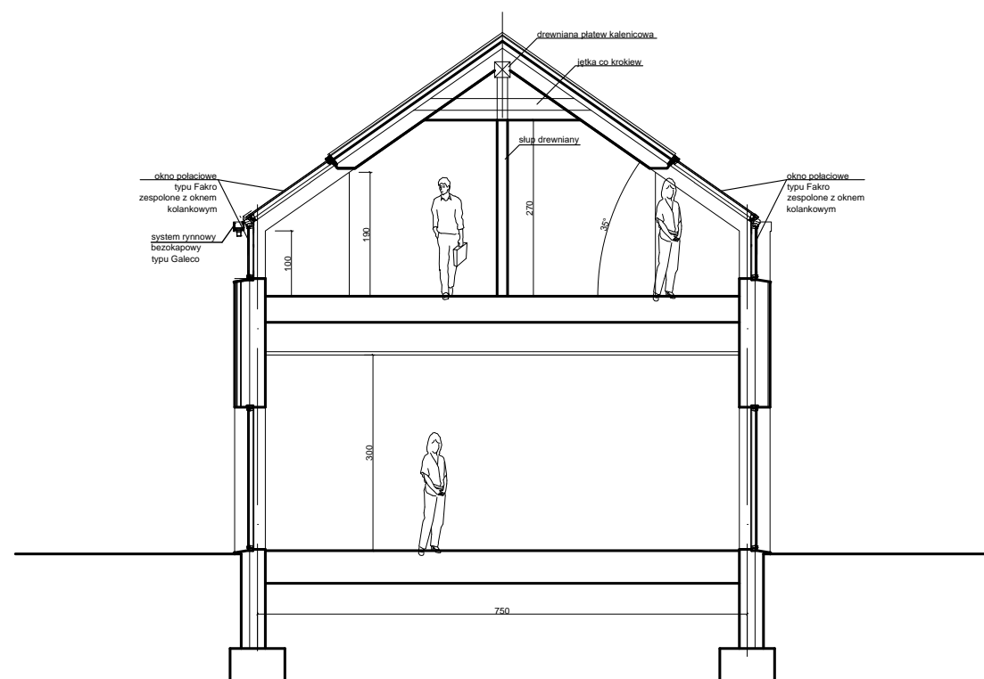
PRZEKRÓJ SCHEMATYCZNY C-C
