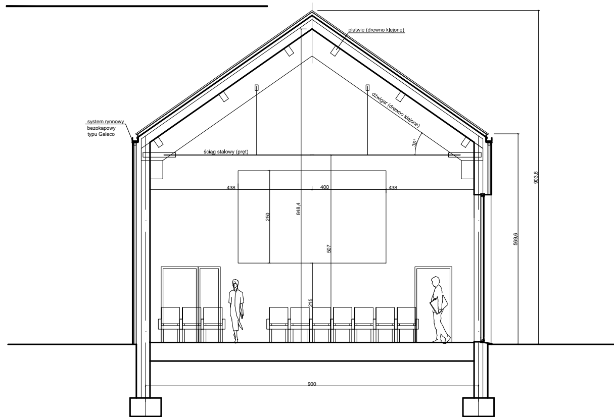
PRZEKRÓJ SCHEMATYCZNY A-A
