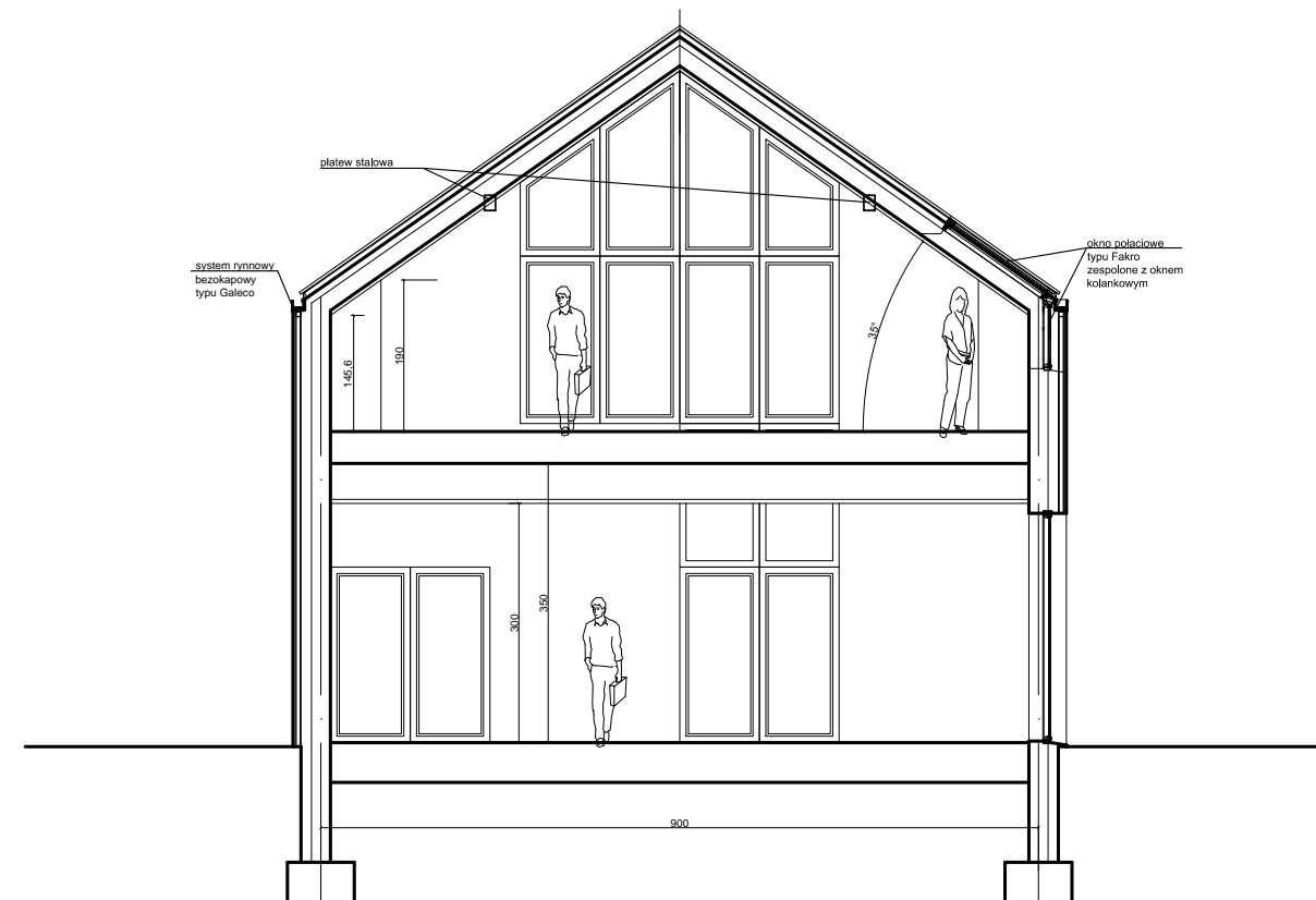
PRZEKRÓJ SCHEMATYCZNY B-B
