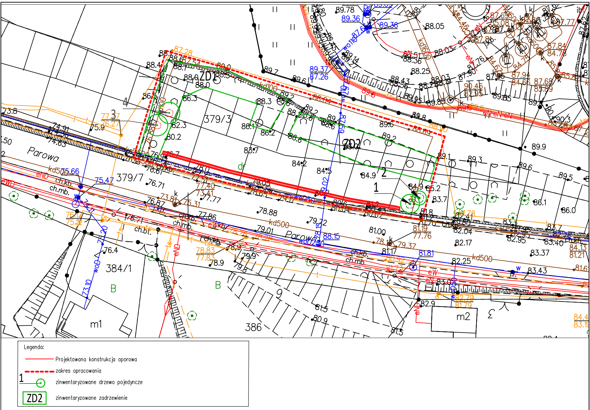
Konstrukcja oporowa wzdłuż ulicy Parowej w Płocku Plan sytuacyjny inwentaryzacja dendrologiczna Rys. 1
