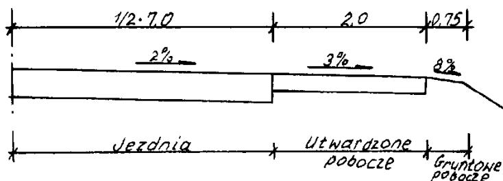
Rys. 2. Przykład utwardzonego pobocza przy etapowaniu rozbudowy szerokości jezdni, wykonanej z betonowej kostki brukowej (wg [20])
