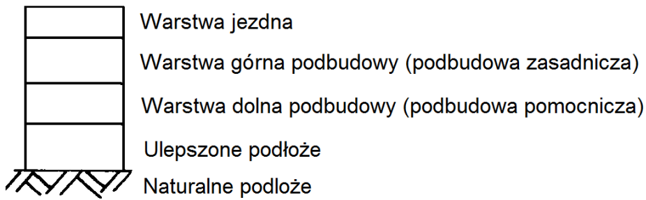
Rys. 3. Konstrukcja nawierzchni utwardzonego pobocza (wg [20])
