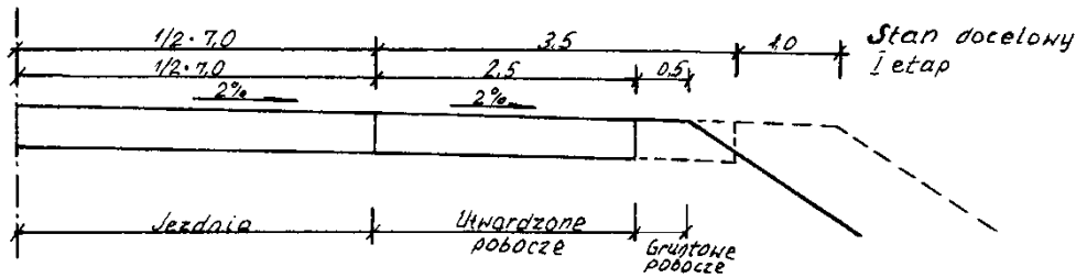
Rys. 3. Konstrukcja nawierzchni utwardzonego pobocza (wg [20])
