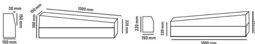
b) krawężnik skośny
