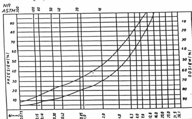
Tablica Nr 13 Wymagania dla mieszanki betonu asfaltowego 0/20 mm półciściego
