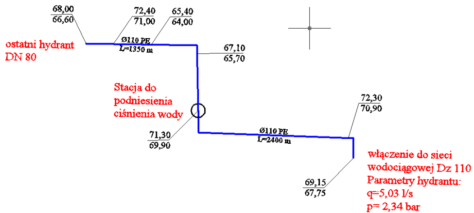
Rys. 2. Schemat wodociągu Klasztorne do m. Strumiennie
