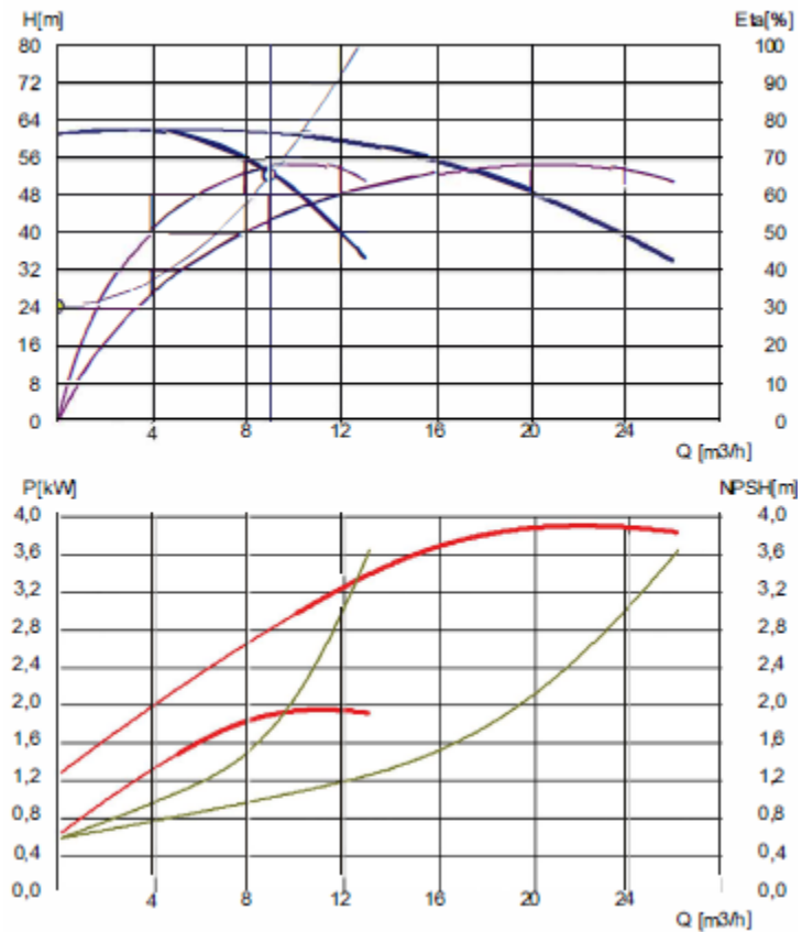
Rys. 1 Wykres pracy jednej pompy H=50,0m.s.l.w Karta katalogowa zestawu pompowego TYP HYDRO-NM 5.B5/11.2 P=2 \times 2,2kW .
