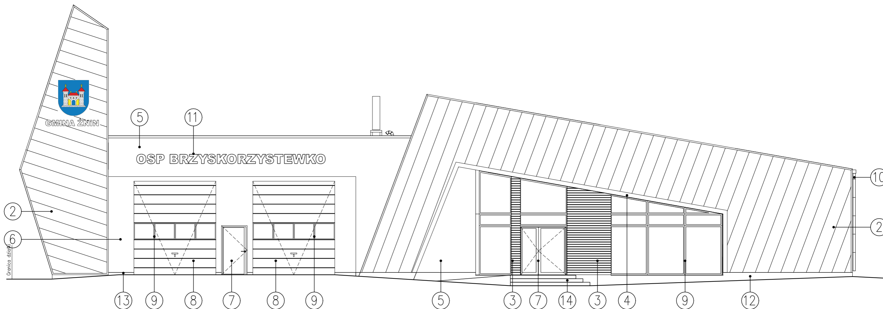
ELEWACJA POŁUDNIOWA
