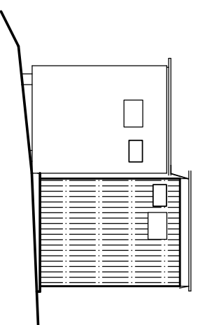
ELEWACJA WSCHODNIA 1:100
