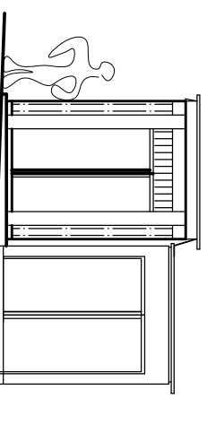
ELEWACJA ZACHODNIA 1:100
