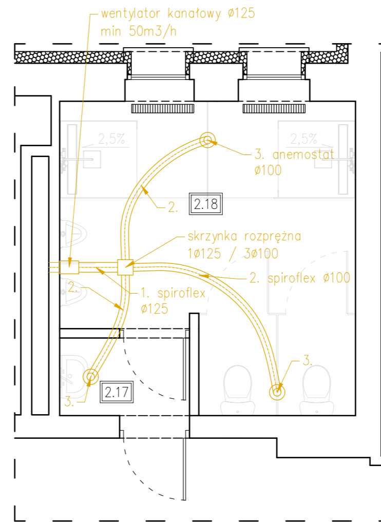
Instalacja wentylacji 1:50
