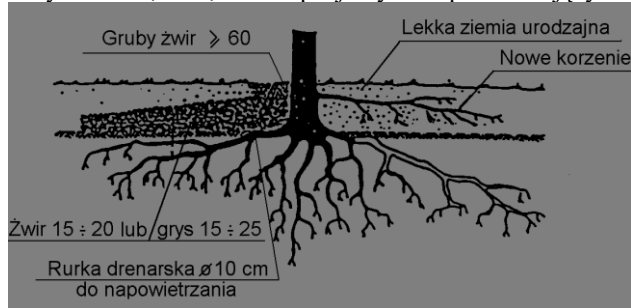
Rys. 5. Studzienka zabezpieczająca pień drzewa przy podwyższeniu terenu powyżej 0,5 m (wg [10])
