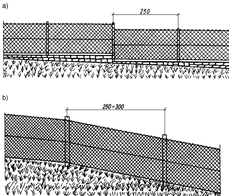
Rys. 6. Przykład ustawienia ogrodzenia siatkowego na terenie pochyłym (wg [6]) a) Ogrodzenie ze stopniami wysokości 25 \div 30 cm (przy spadku terenu od 1:16 do 1:30) b) Ogrodzenie równoległe do terenu
