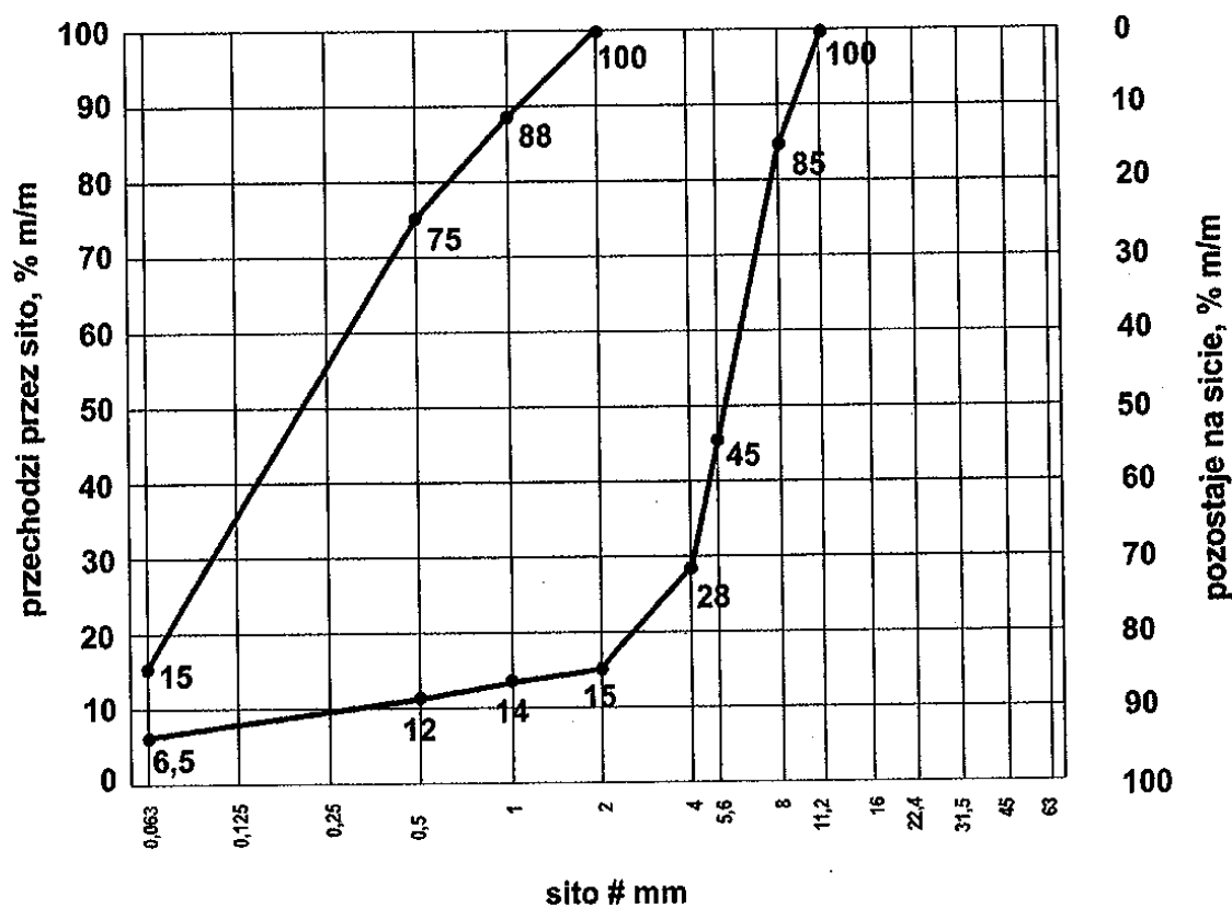
Rys. .1.2 Uziarnienie mieszanki CBGM 0/8
