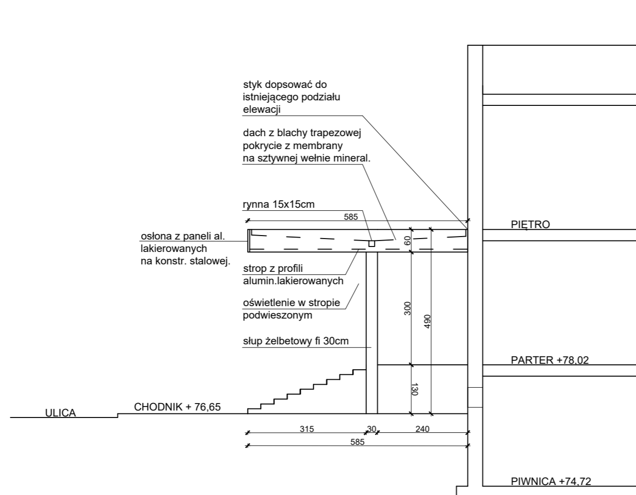
SCHEMAT PRZEKROJU 1:100
