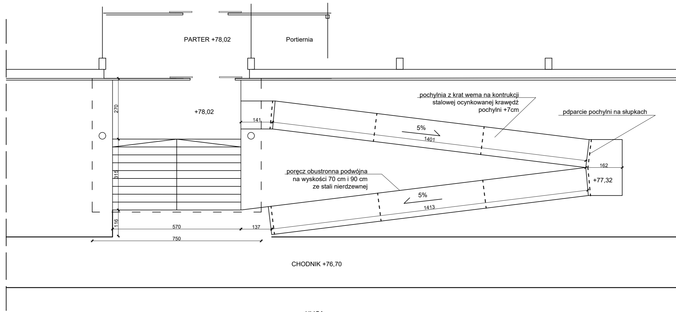
RZUT WEJŚCIA 1:100
