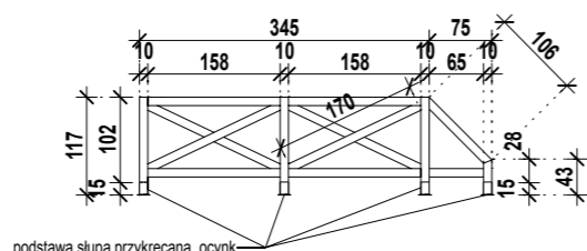
Profil balustrady: 10x10cm, drewno lite iglaste
