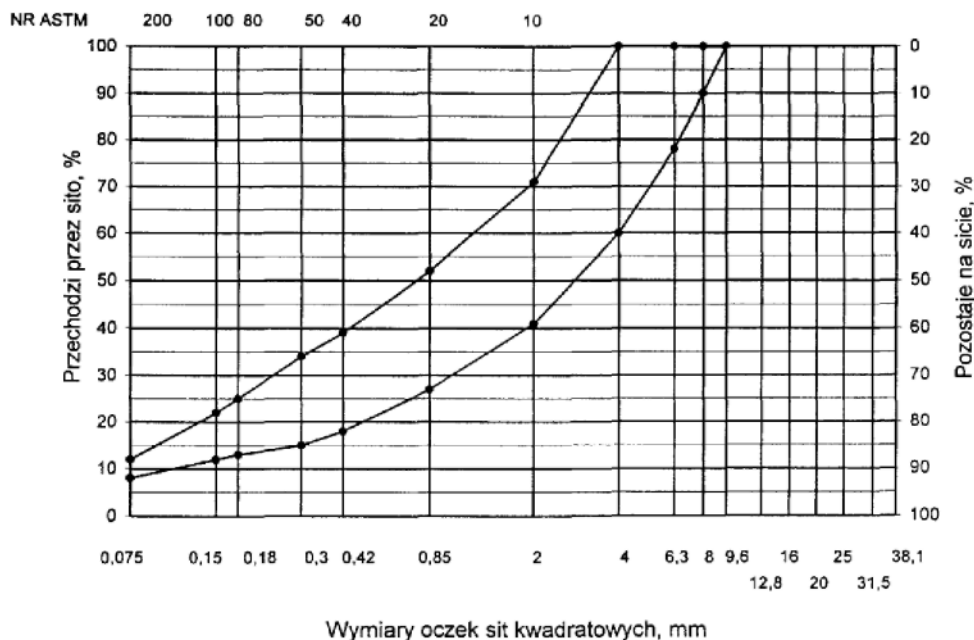
Rys. 2. Krzywe graniczne uziarnienia mieszanki mineralnej BA od 0 do 8 mm, od 0 do 6,3 mm do warstwy ściernalnej nawierzchni drogi o obciążeniu mchem nawierzchni drogi o obciążeniu ruchem KR1 lub KR2
