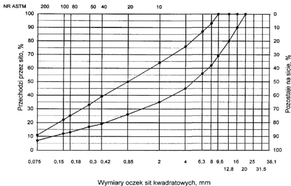
Rys. 2. Krzywe graniczne uziarnienia mieszanki mineralnej BA od 0 do 8 mm, od 0 do 6,3 mm do warstwy ściernalnej nawierzchni drogi o obciążeniu mchem nawierzchni drogi o obciążeniu ruchem KR1 lub KR2
