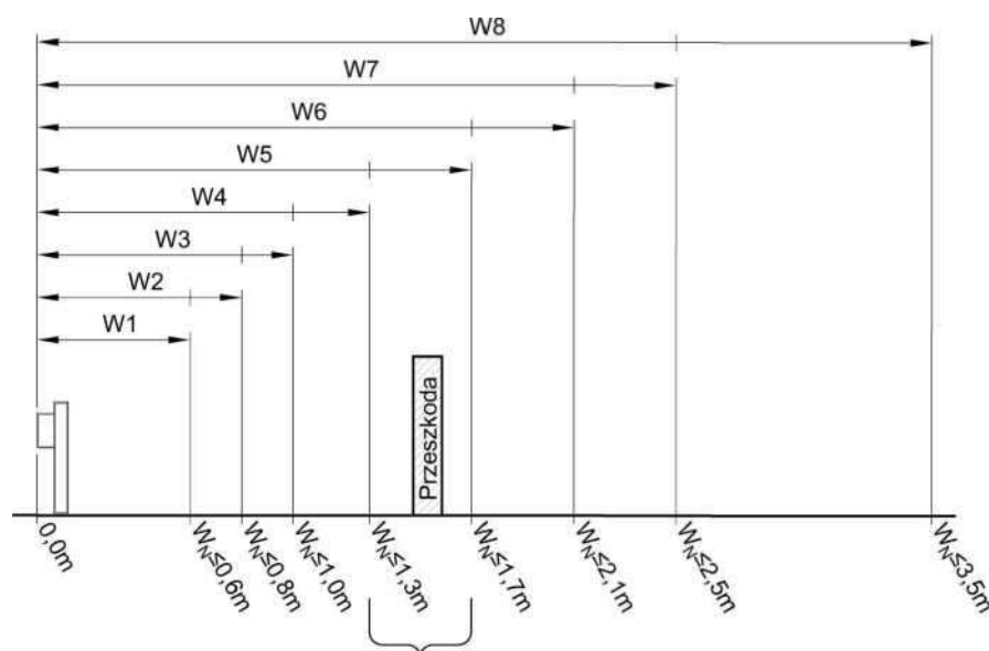
Przedział szerokości pracującej bariery dla klasy W5, który spełnia wymagania zabezpieczenia pojazdu przed najechaniem na przeszkodę położoną w zakresie odległości 1,3 < WN \leq 1,7 m. (zasada dotyczy wszystkich klas szerokości pracującej)
