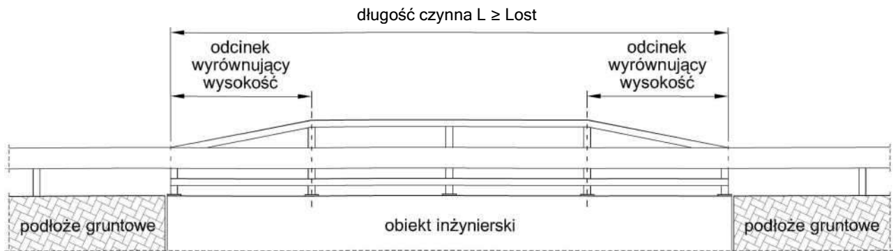
Rys. 12. Czynna długość bariery na obiekcie inżynierskim uwzględniająca odcinek wyrównujący wysokość barier.
