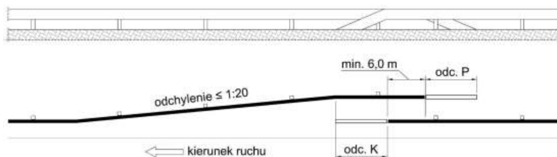
Rys. 19. Schemat zastosowania przerwy w barierze ochronnej.
