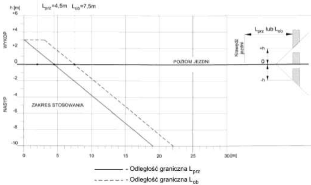
Rys. 1. Odległości graniczne stosowania barier ochronnych dla dróg o prędkości V_{dp} \leq 90 km/h.
