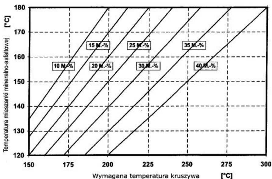
Tablica 13. Temperatura kruszywa w zależności od ilości zimnego i suchego granulaku
