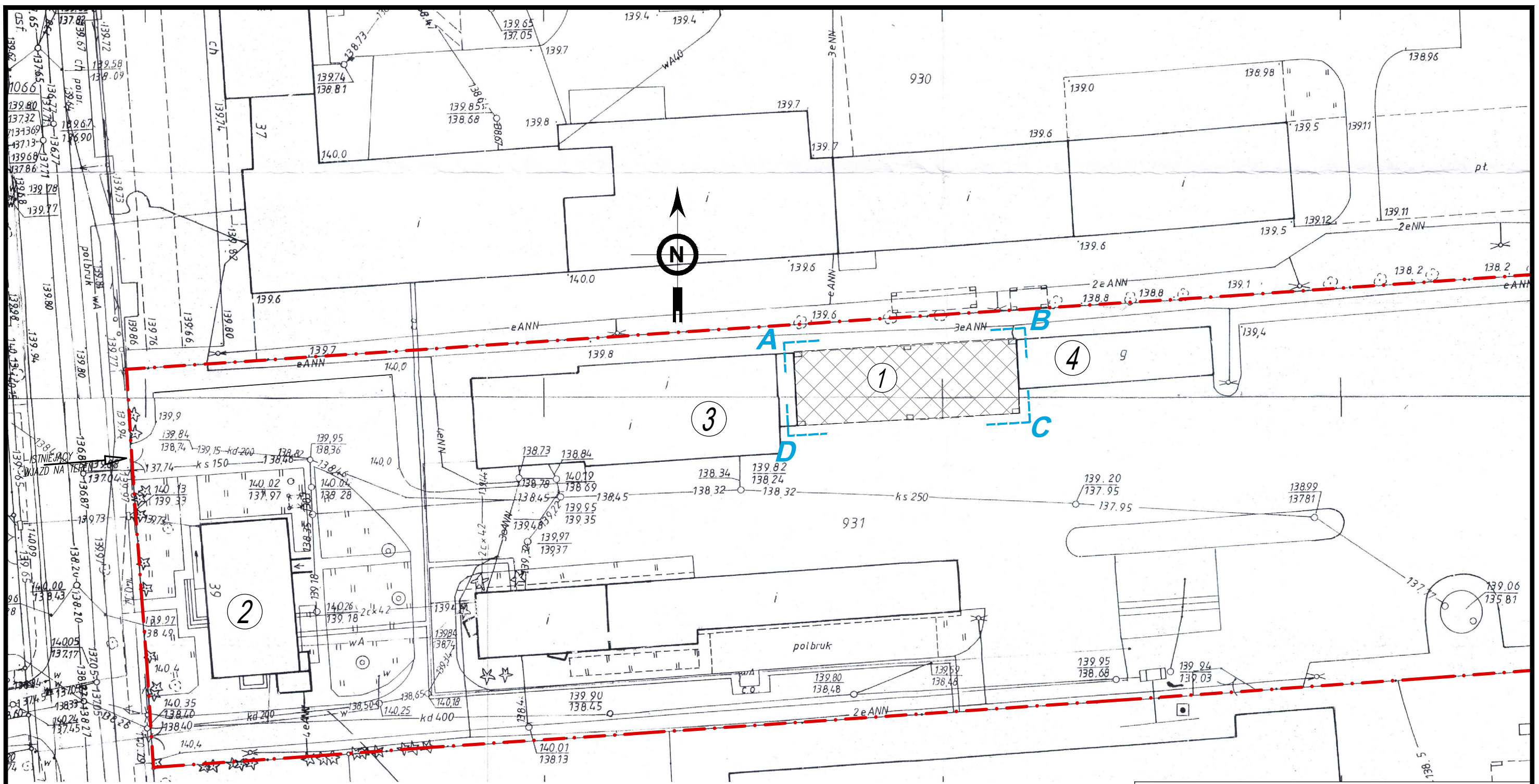
PLAN SYTUACYJNY. skala 1:500
