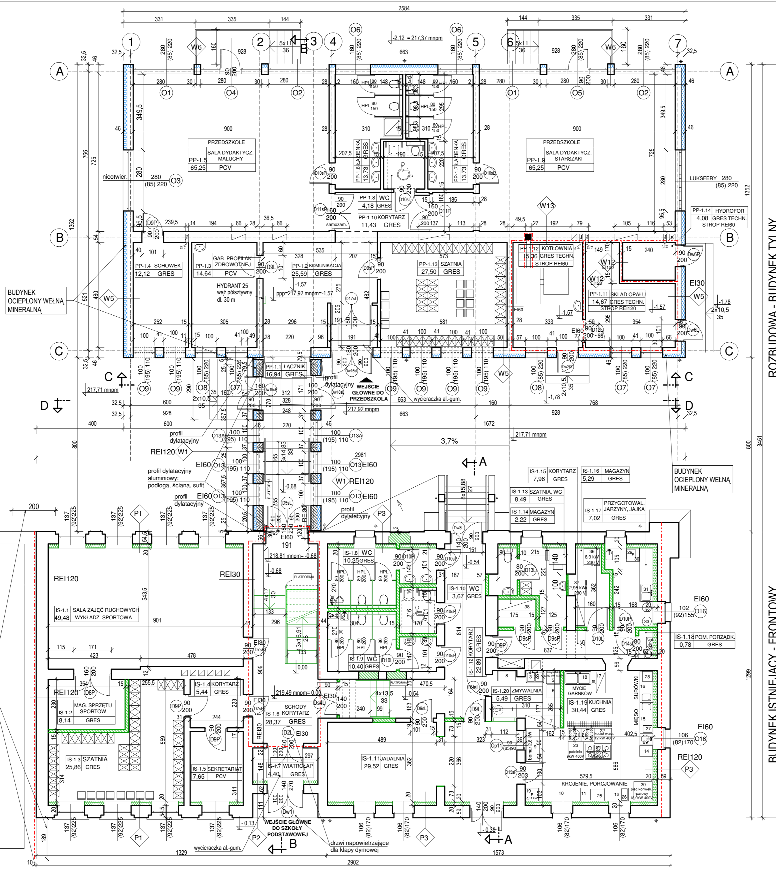
ZESTAWIENIE POMIESZCZEŃ PARTERU
