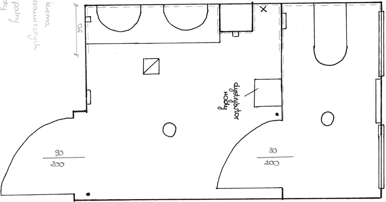
006 - WC DAMSKIE
