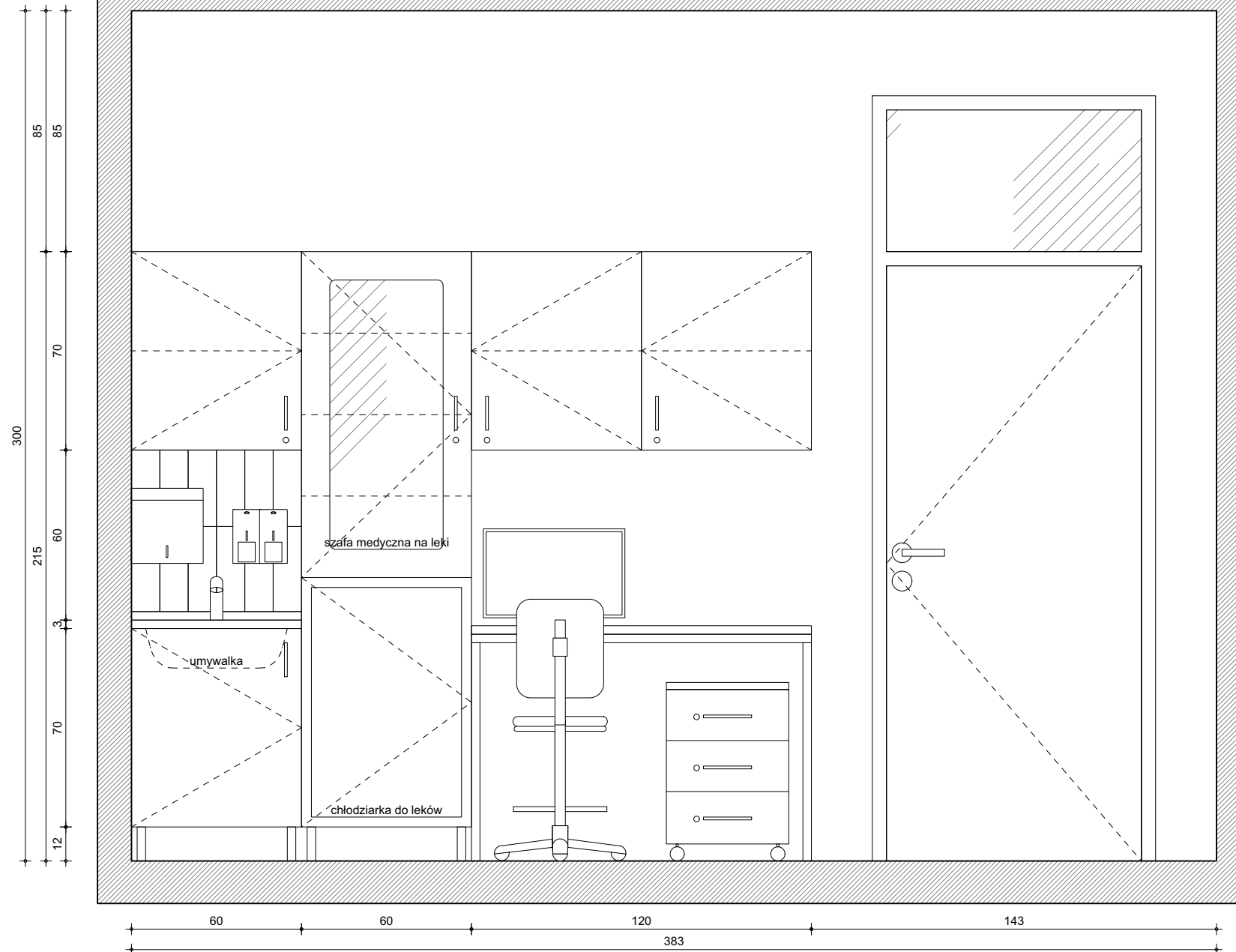
WIDOK Z PRZODU
