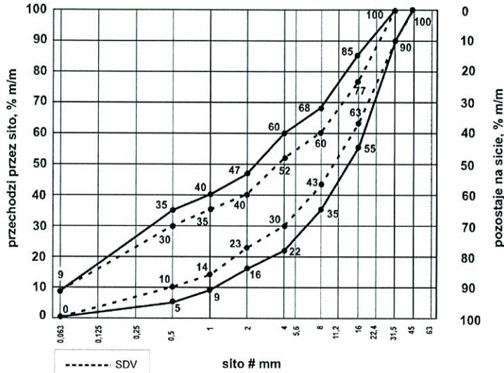
Rys.1. Uziarnienie mieszanki niezwiązanej 0/31,5 dla podbudowy zasadniczej
