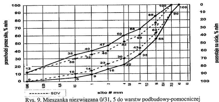
Rys. 9. Mieszanka niezwiązana 0/31, 5 do warstw podbudowy-pomocniczej
