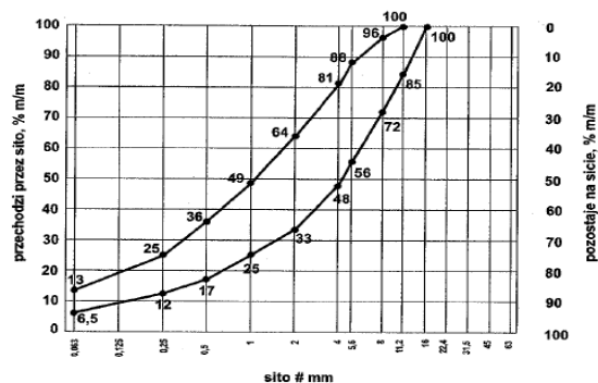
Rys. 1 Uziarnienie mieszanki CBGM 0/11,2
