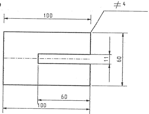
Blacha uszczelniająca ciągnio wewnętrznie 1:2 (13)
