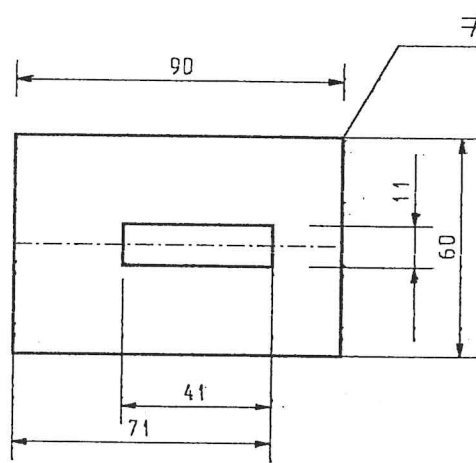
Blacha uszczelniająca ciągnio zewnątrznie 1:2 (12)
