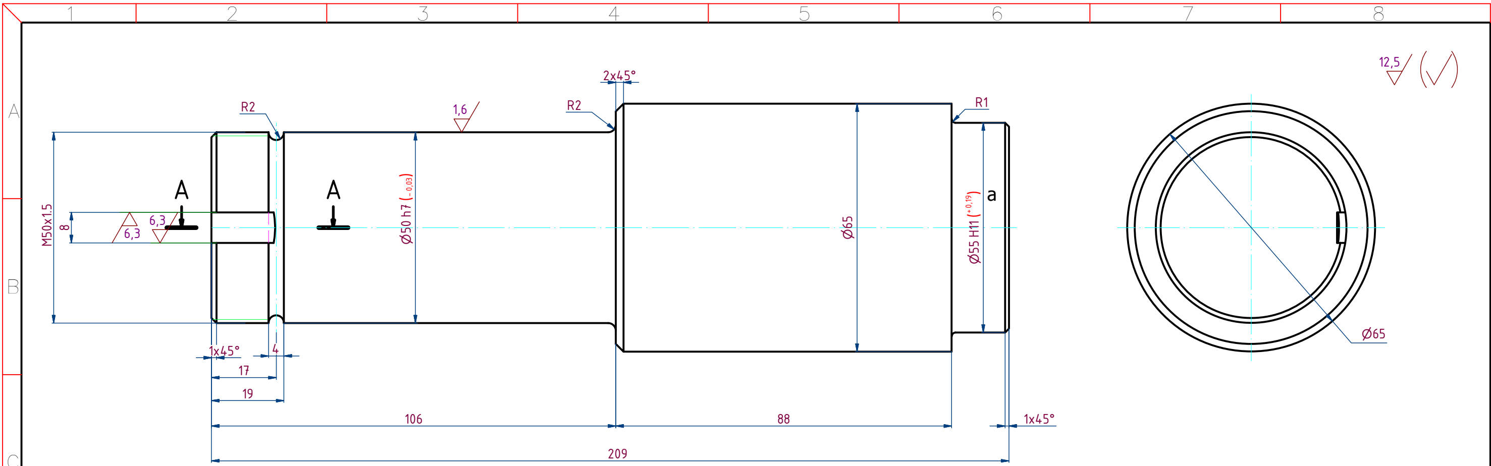
A-A (1:1)
