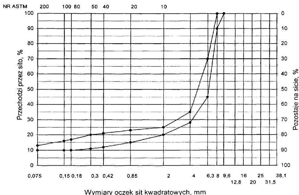
Rys. 7. Krzywe graniczne uziarnienia mieszanki mineralnej SMA od 0 do 8 mm do warstwy ścieralnej nawierzchni drogi
