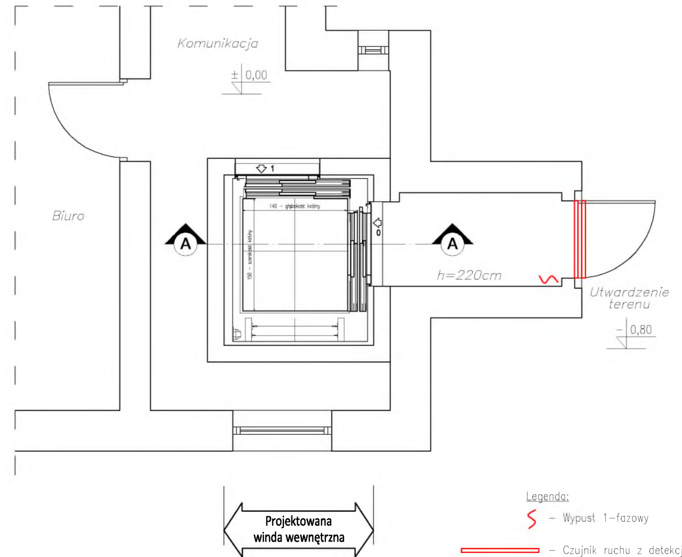
Rzut parteru
