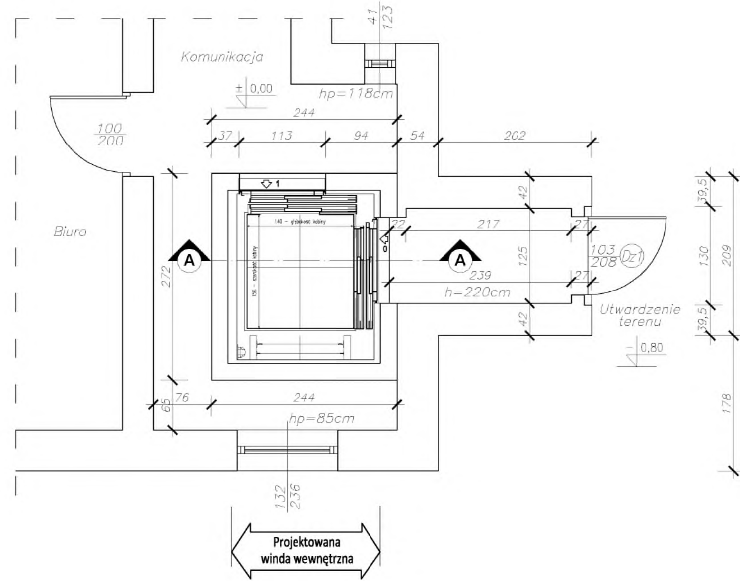
Rzut parteru
