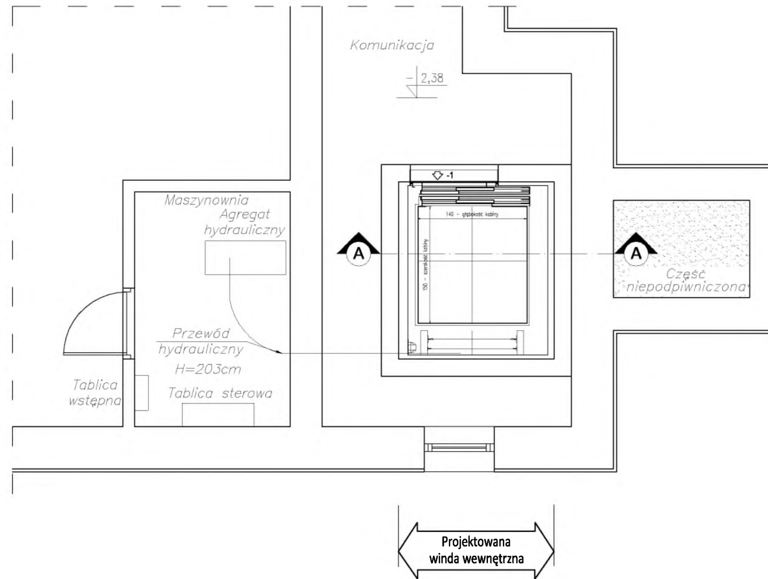
Rzut piwnicy
