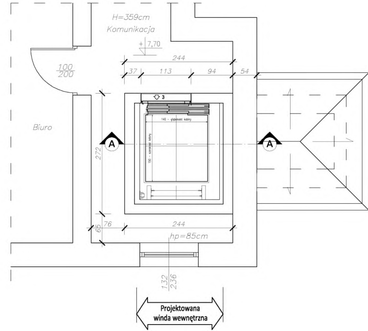
Rzut II piętra
