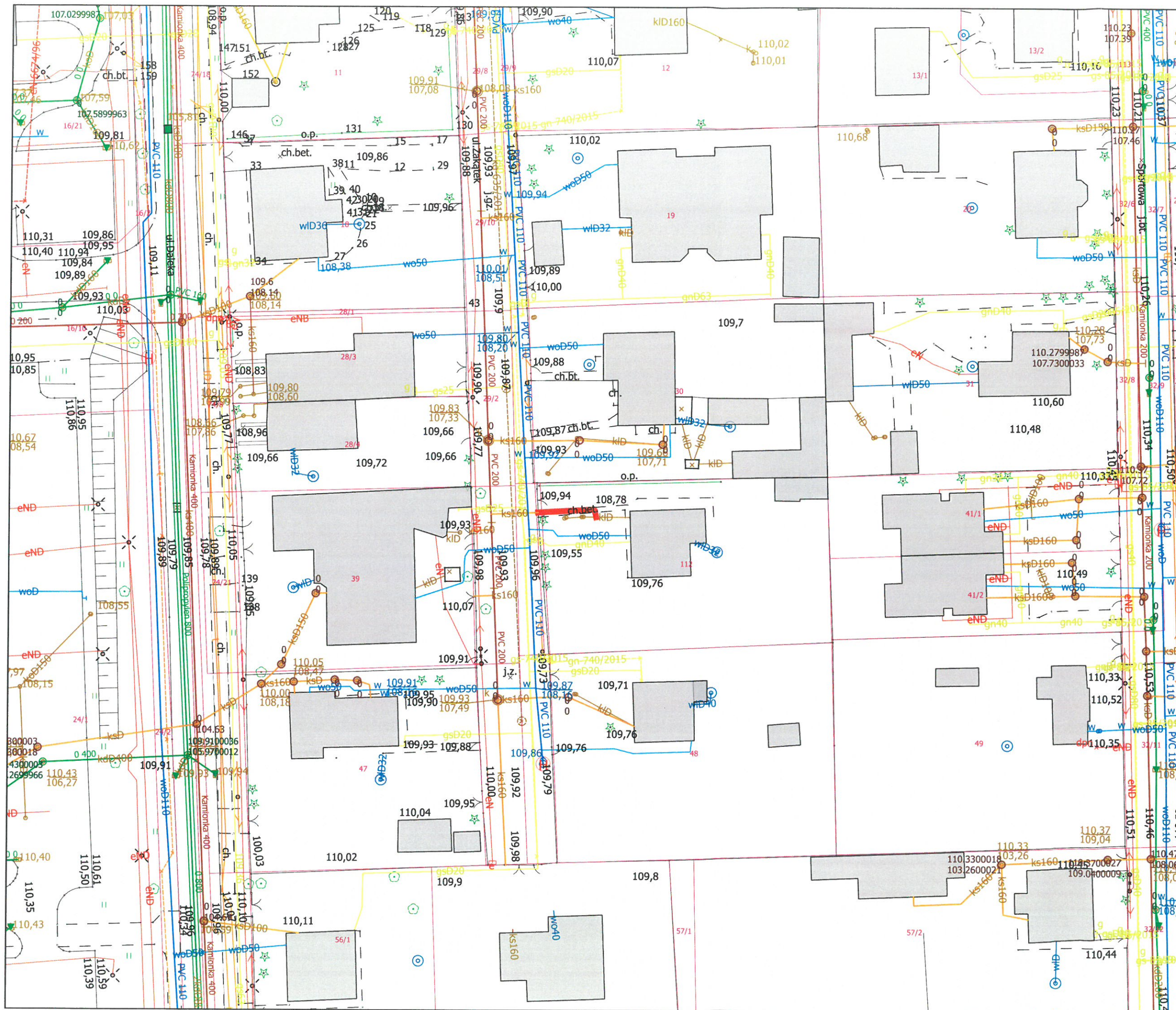
Przyłącze kanalizacji sanitarnej Adres: ul. Zakątek 6 Grodzisk Mazowiecki dz. nr ew. 112 obręb 58
