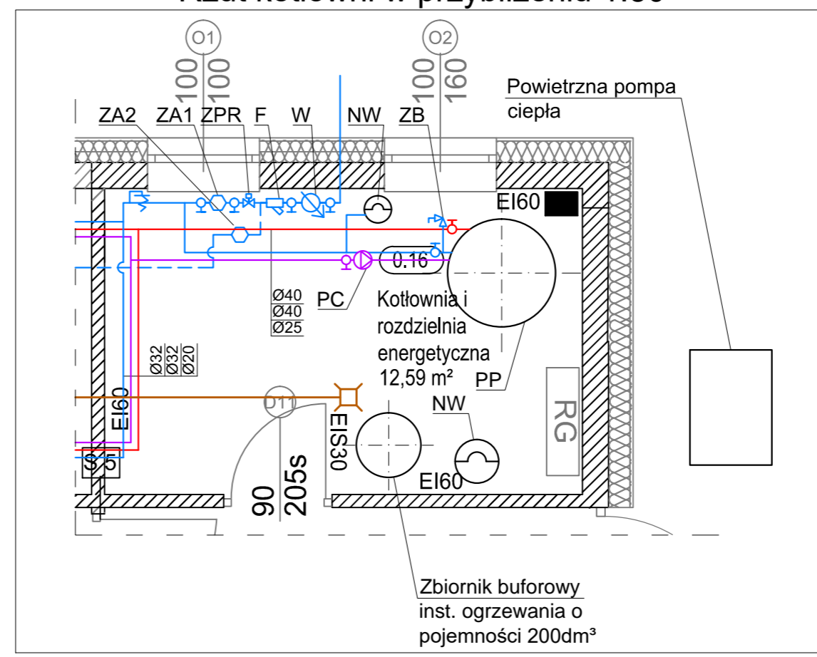
Rzut kotłowni w przybliżeniu 1:50
