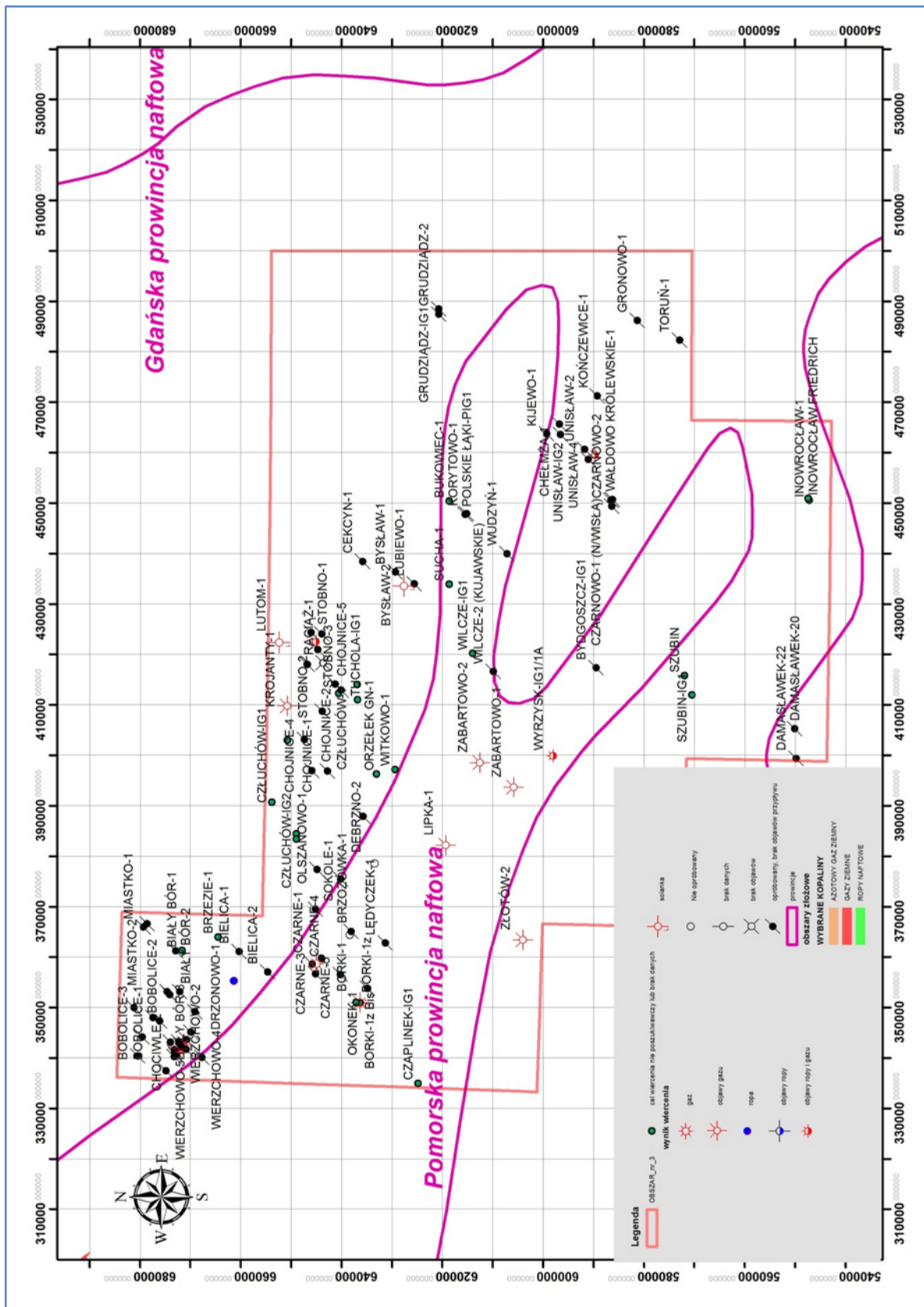
Fig. 2 Głębokie otwory odwiercone na wyznaczonym obszarze wg. PGNiG.
