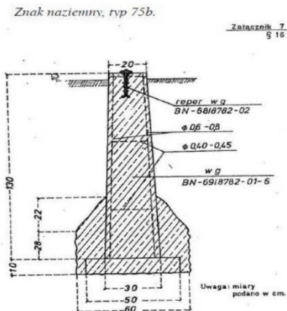
Rys.3 ZNAK WYSOKOŚCIOWY NAZIEMNY - typ 75 b Słup betonowy na płycie z poduszką - 140
