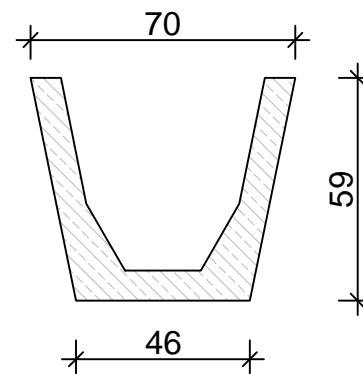
Korytko odwodnieniowe - kolejowe 70/46x59x50cm
