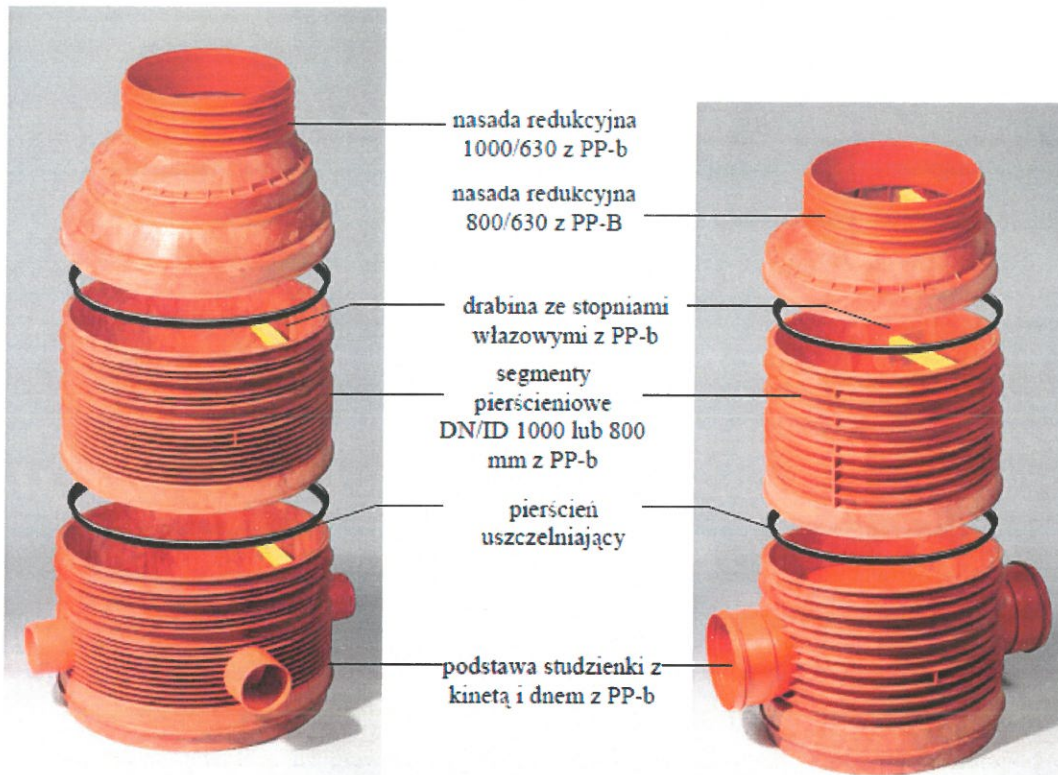
Rys. 2 Studzienka PRO 1000
