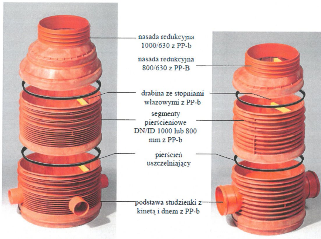
Rys.3 Studzienka PRO 800
