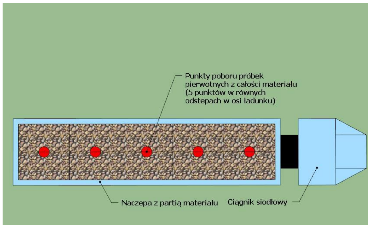
Pobieranie próbek pierwotnych z naczepy pojazdu
