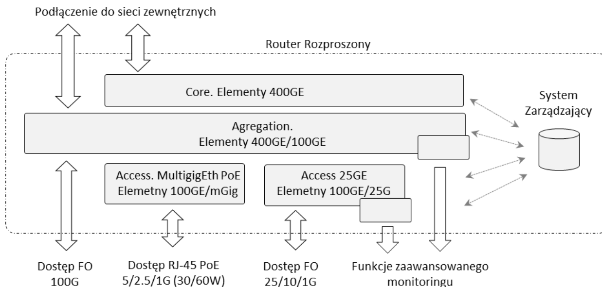
Rysunek 1 Schemat funkcjonalny routera rozproszonego
