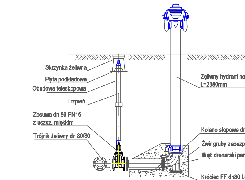
Schemat montażu hydrantu nadziemnego
