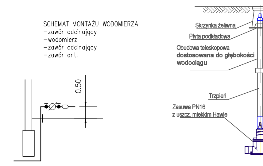
Schemat montażu zasowy
