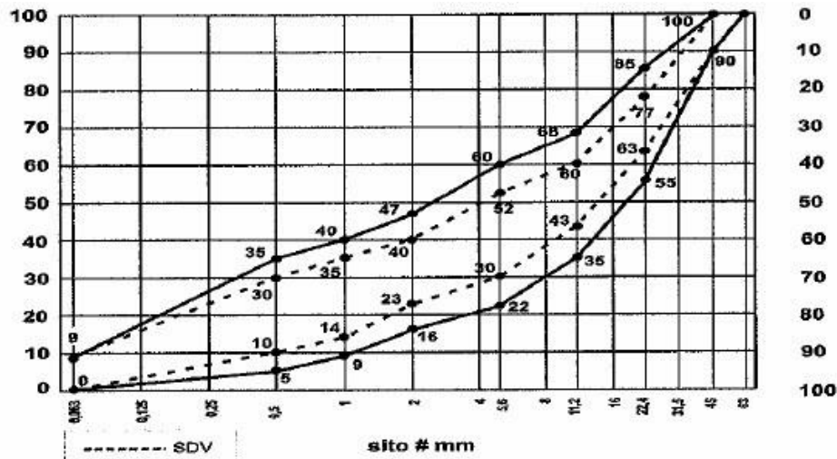
Rys. 11. Krzywe graniczne uziarnienia mieszanki niezwiązanej 0/31,5 mm do podbudowy zasadniczej
