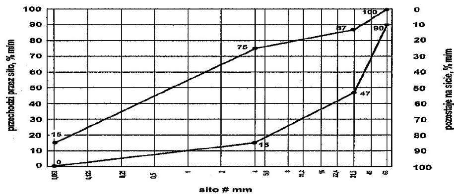
Rys. 6. Krzywe graniczne uziarnienia mieszanki kruszyw 0/45 mm do górnej warstwy podłoża ulepszzonego
