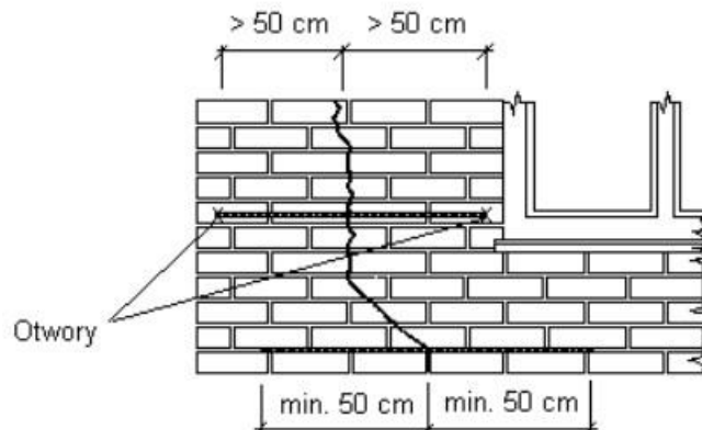
Przykładowy szkic zszywania pęknięć ściany
