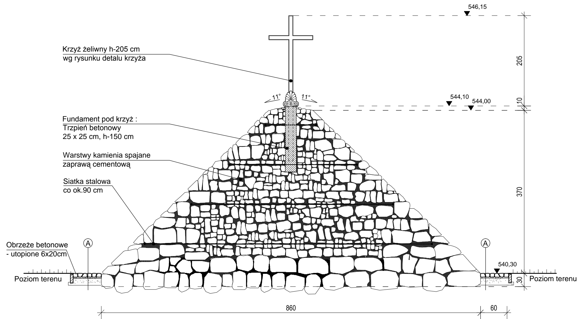
PRZEKRÓJ A-A SKALA 1:50
