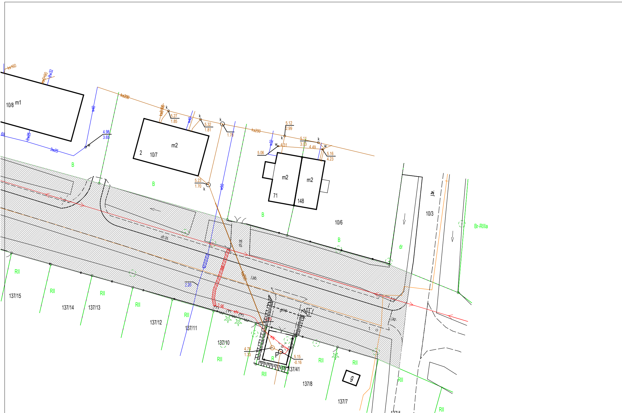
PRZEBUDOWA DRÓGI GMINNEJ WEWNĘTRZNEJ W BOREŃTACH DRUGICH W GMINIE LICHNOWY - PRZEWIDYWANY ZAKRĘS OPRACOWANIA 4/4
