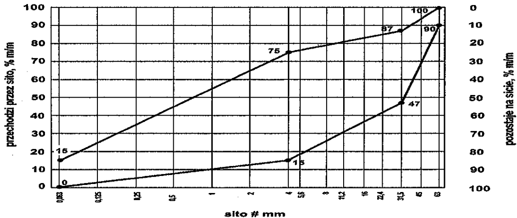
Rys. 7. Krzywe graniczne uziarnienia mieszanki kruszywo 0/63 mm do górnej warstwy podłoża ulepszanego
