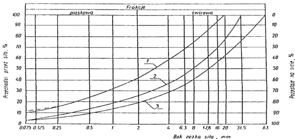
Rysunek 1. Pole dobrego uziarnienia kruszyw przeznaczonych na warstwy ulepszonych podłoża i podbudowy wykonywanych metodą stabilizacji mechanicznej
