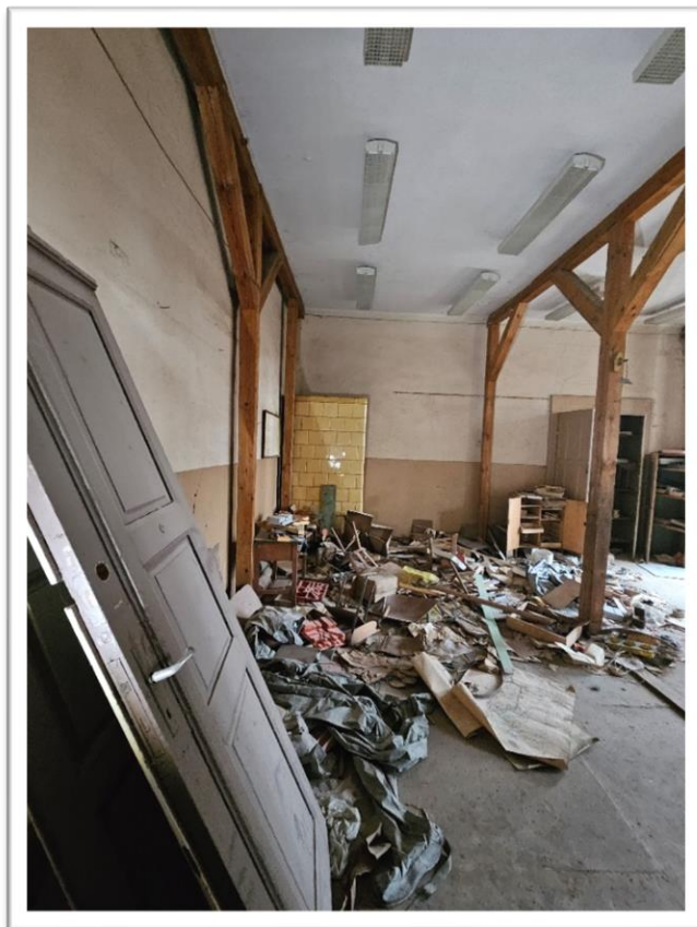
Fotografia 26 Stan istniejący (inwentaryzacja pom. 03 parter) wschód – Czytelnia – podparcie stropu.
