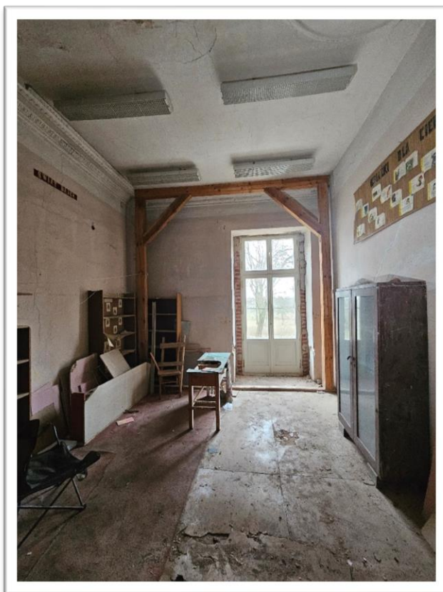
Fotografia 21 Stan istniejący (inventaryzacja pom. 04 parter) północ – Biblioteka – podparcie stropu.
