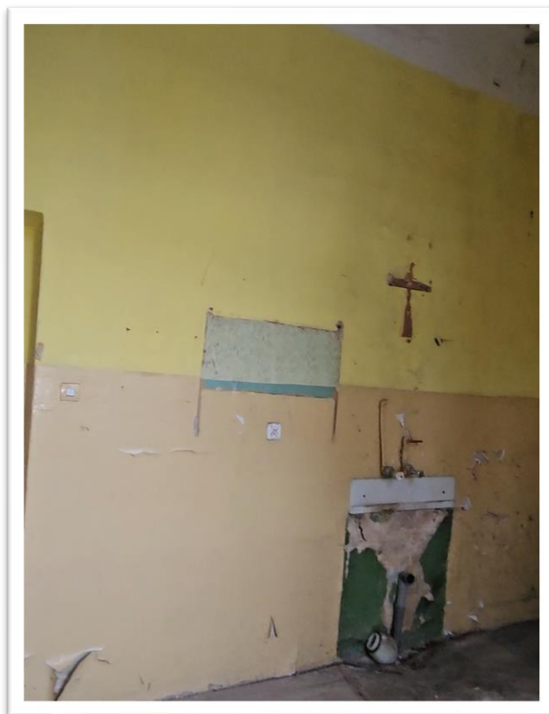
Fotografia 46 Stan istniejący (inventaryzacja pom. 21 parter) – Zaplecze socjalne – widok stanu po adaptacji pomieszczeń na przedszkole.
