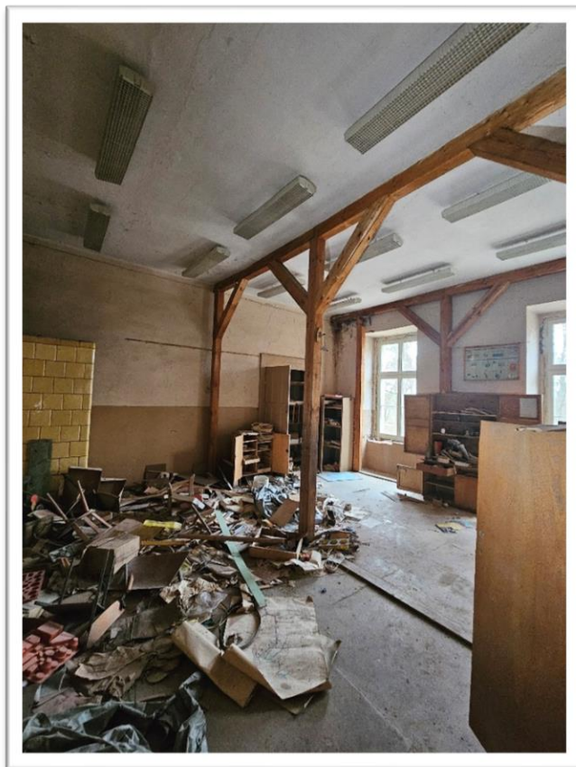
Fotografia 27 Stan istniejący (inwentaryzacja pom. 03 parter) południe, wschód – Czytelnia – podparcie stropu.
