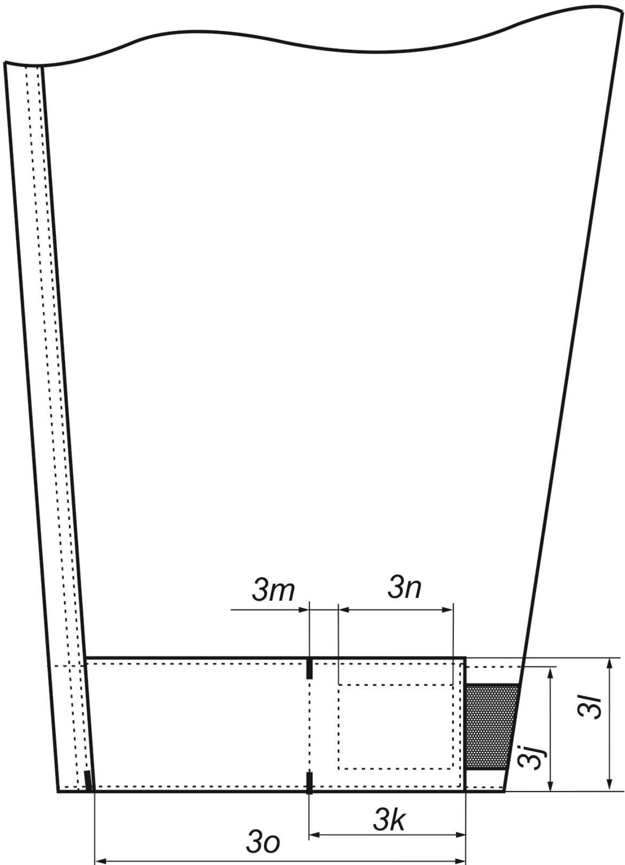
Rysunek 12 – bluza dół rękawa
