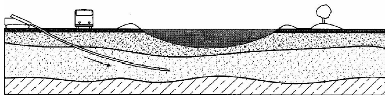
Rys. 1) Przewiert pilotażowy
