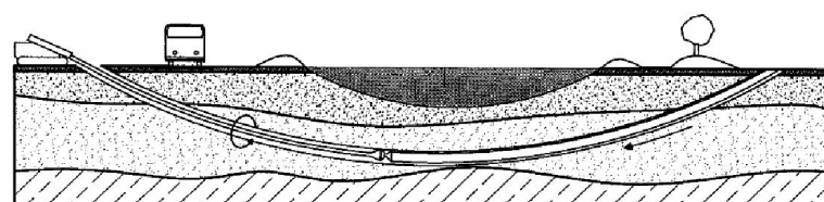
Rys. 3) Przeciąganie rurociągu
