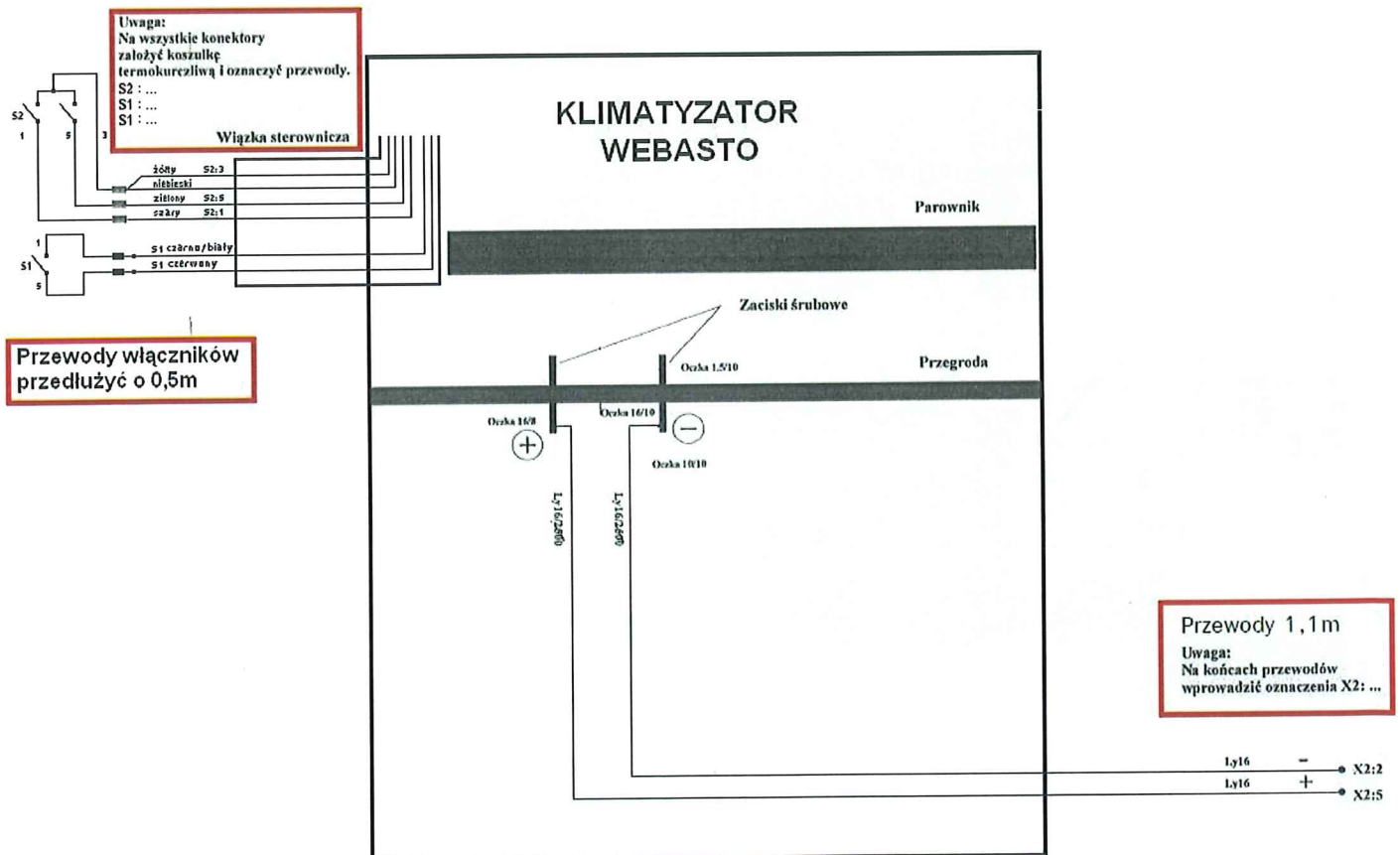
Rys. 1 Modyfikacje dostosowujące klimatyzator
