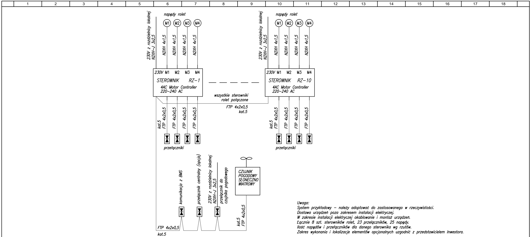
SCHEMAT STEROWANIA ROLETAMI
