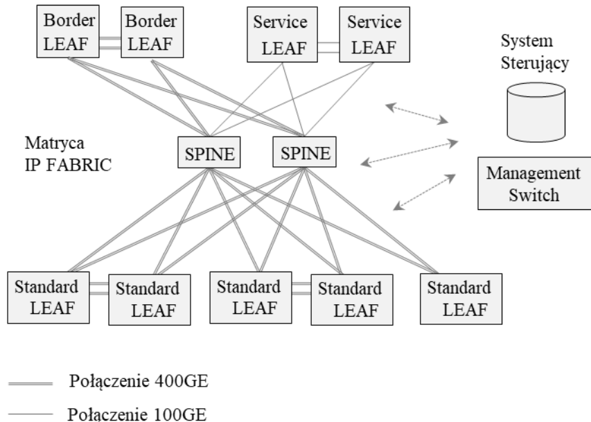
Rysunek 2 Schemat funkcjonalny Systemu Przetwarzania Pakietowego
