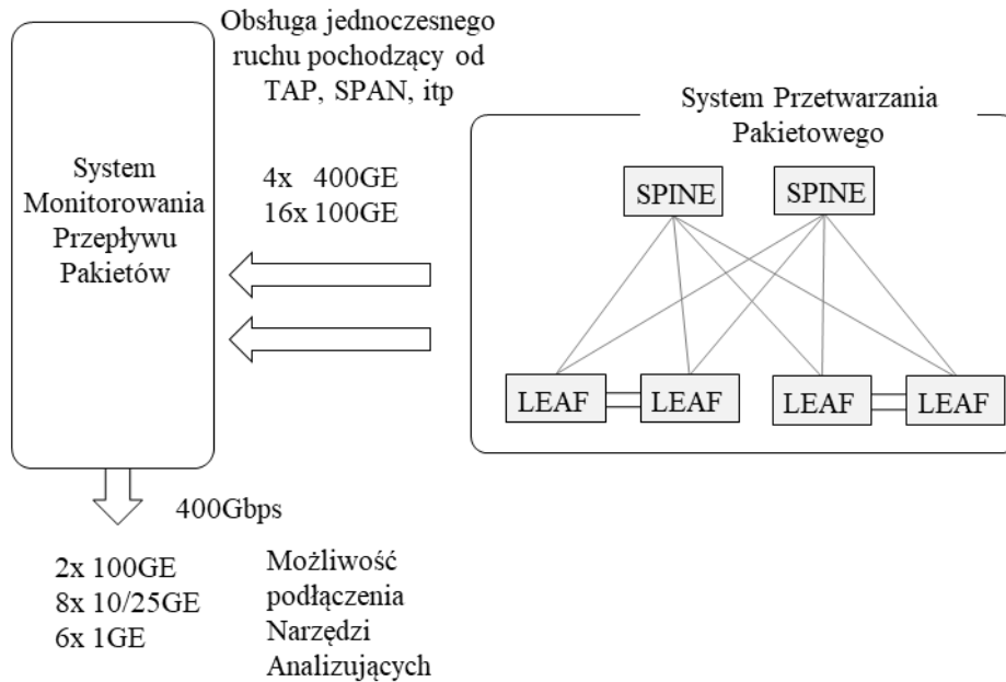
Rysunek 3 Schemat funkcjonalny Systemu Monitorowania Przepływów
