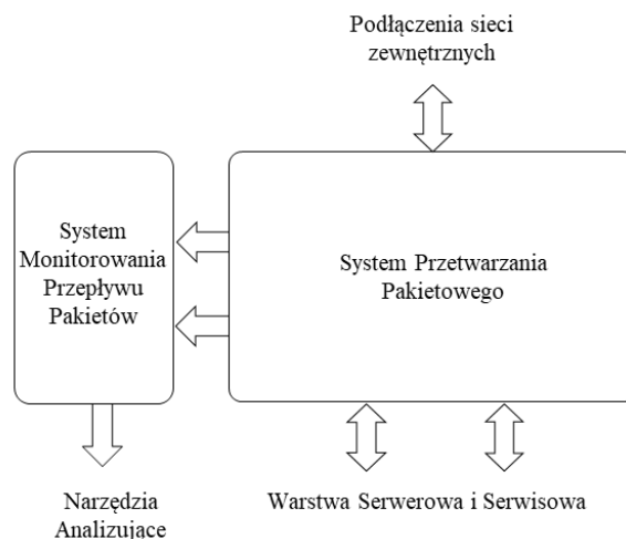
Rysunek 1 Schemat funkcjonalny routera rozproszonego
